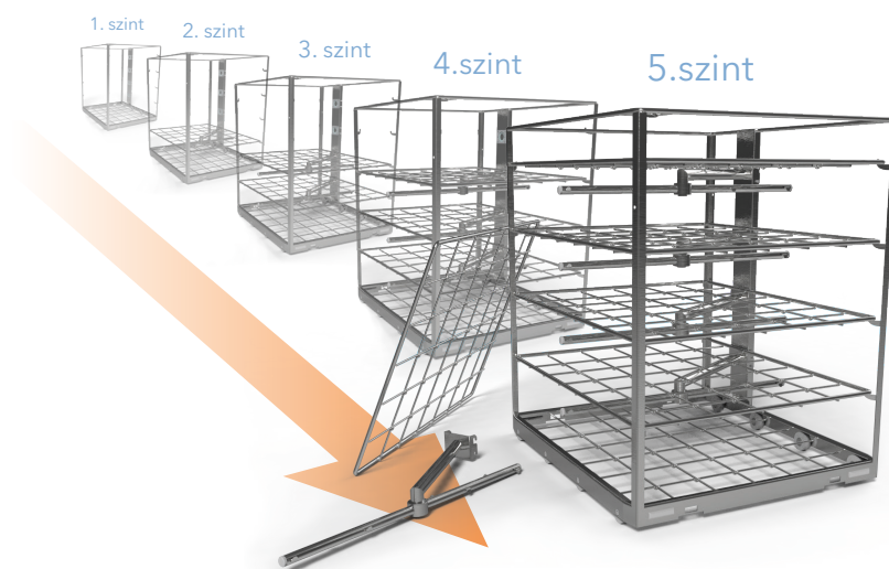
5 szintes szabadon állítható állvány
